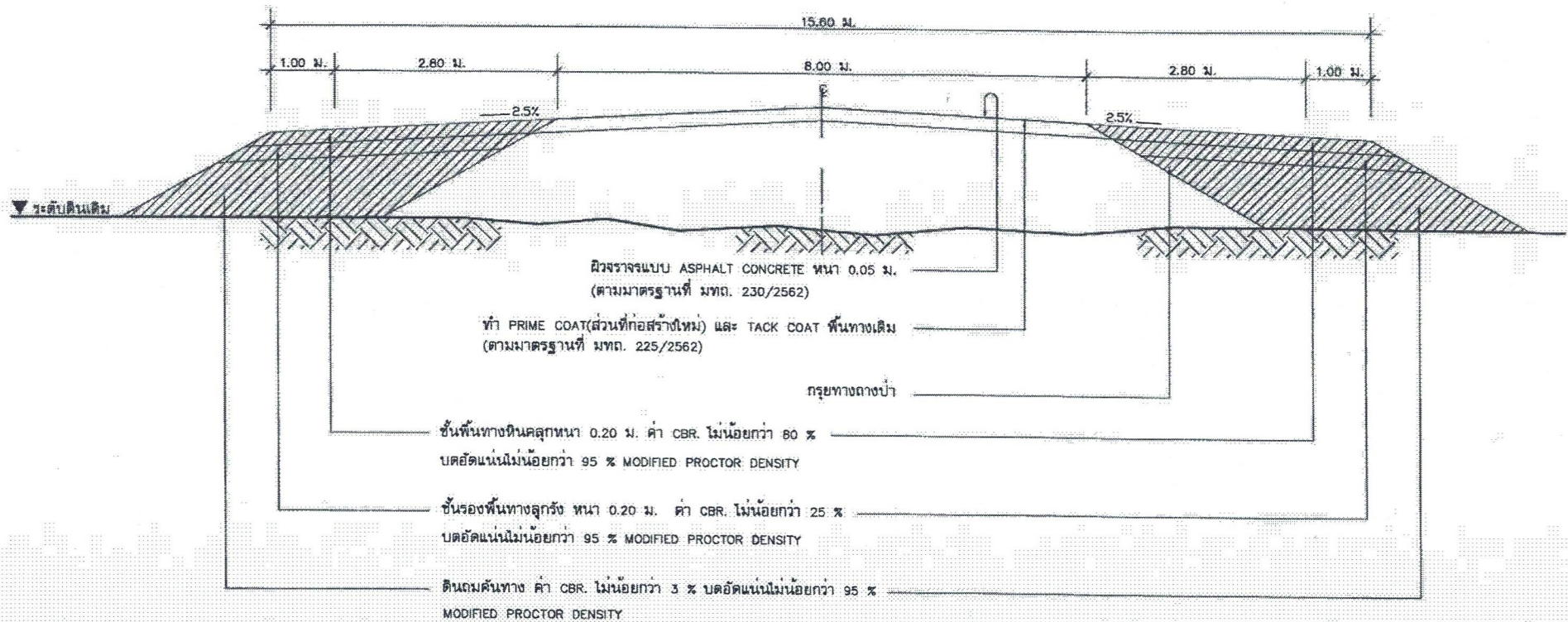
รูปตัดโครงสร้างทางผิวจราจรแบบ ASPHALT CONCRETE มาตรฐาน 1 : 75
