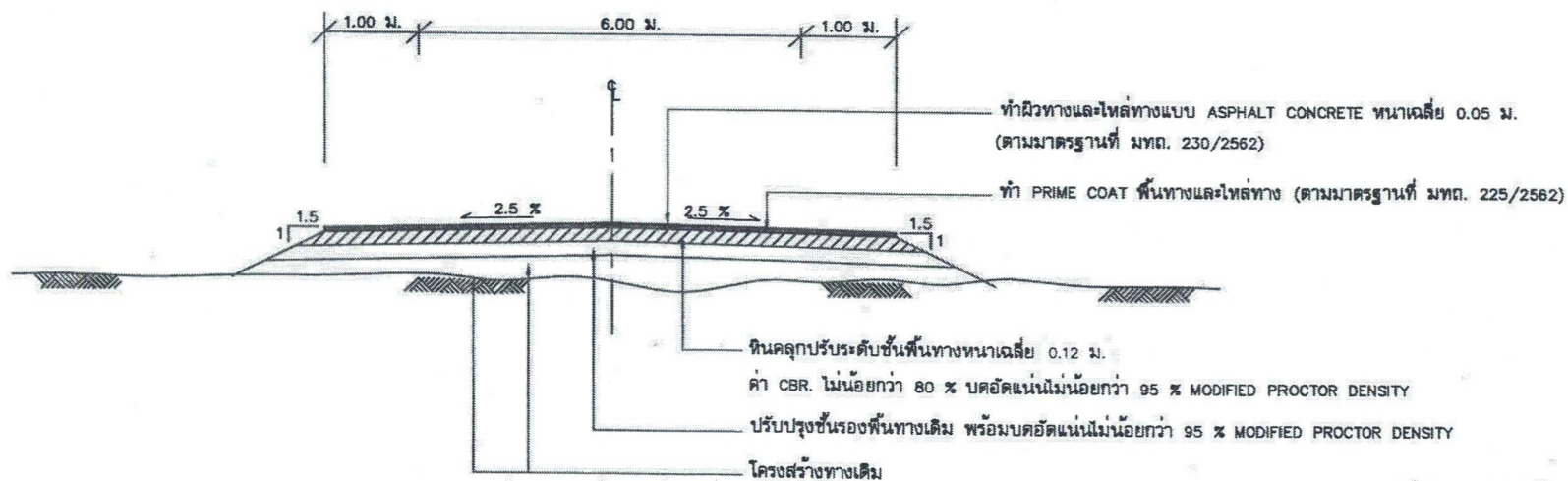
รูปตัดโครงสร้างทางผิวจราจรแบบ ASPHALT CONCRETE และ กม.ที่ 5+000 ถึง กม.ที่ 6+400
