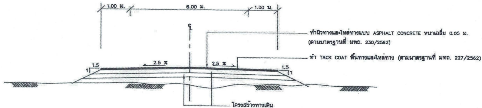
รูปตัดโครงสร้างทางผิวจราจรแบบ ASPHALT CONCRETE กม.ที่ 0+000 ถึง กม.ที่ 0+400
