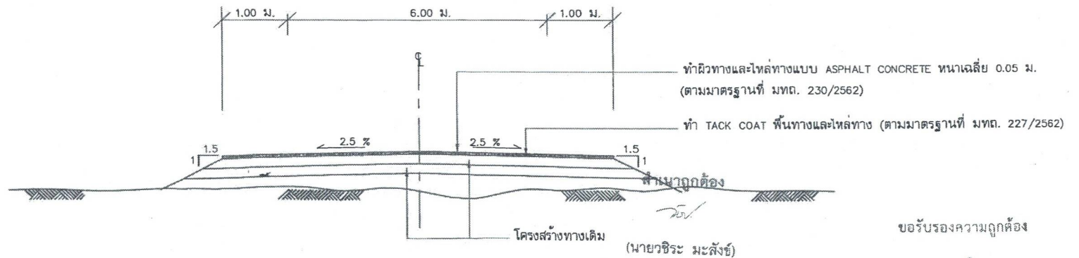
รูปตัดโครงสร้างทางผิวจราจรแบบ ASPHALT CONCRETE กม.ที่ 3+350 ถึง กม.ที่ 3+850
