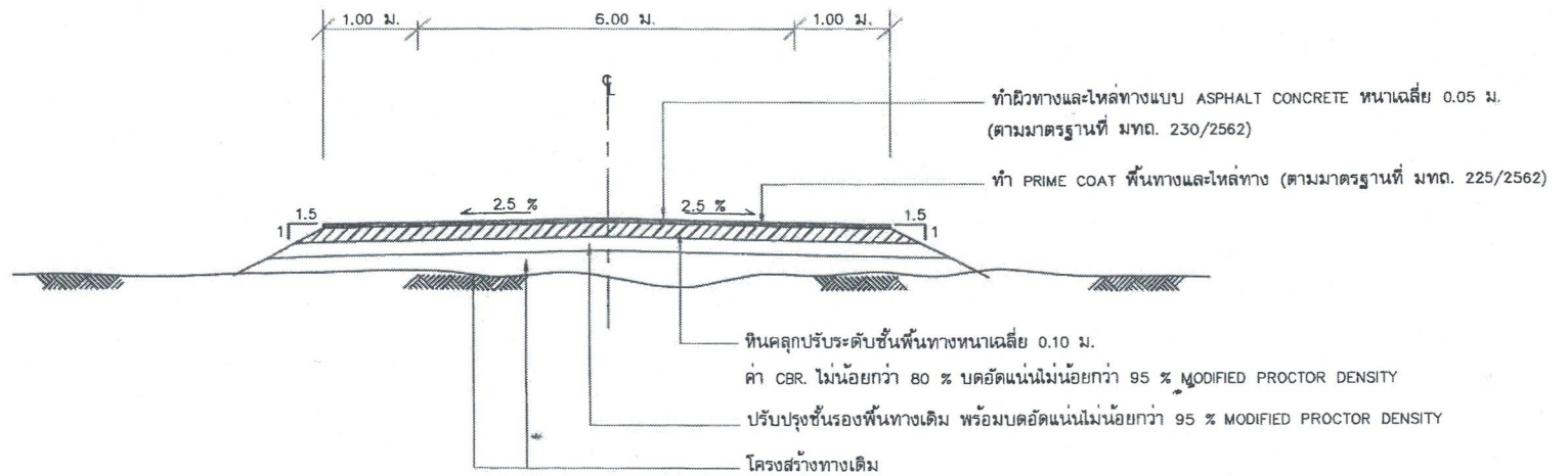
รูปตัดโครงสร้างทางผิวจราจรแบบ ASPHALT CONCRETE กม.ที่ 2+000 ถึง กม.ที่ 2+300 และ กม.ที่ 2+760 ถึง กม.ที่ 3+350
