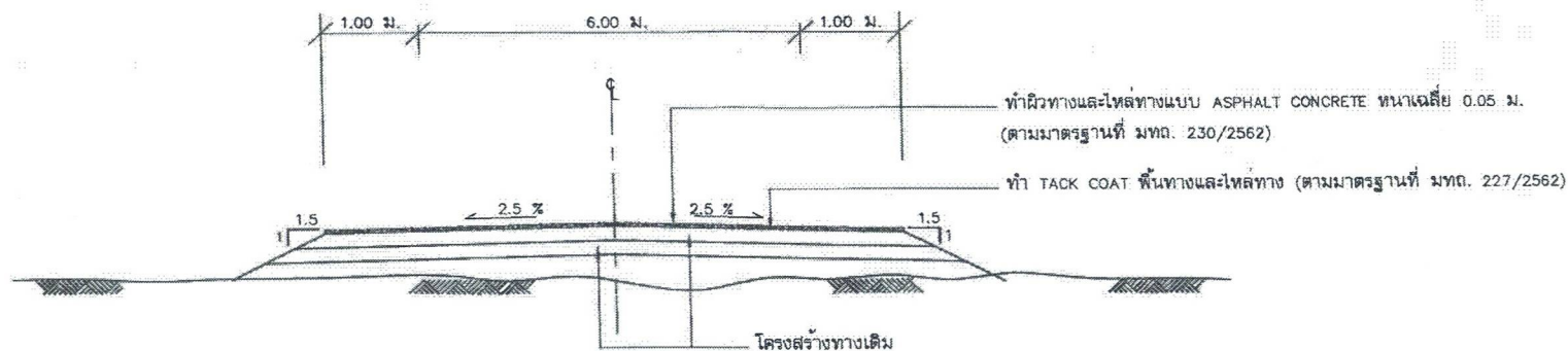
รูปตัดโครงสร้างทางผิวจราจรแบบ ASPHALT CONCRETE กม.ที่ 0+000 ถึง กม.ที่ 0+560
