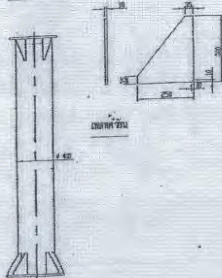
แบบขยายเสาเข็ม
