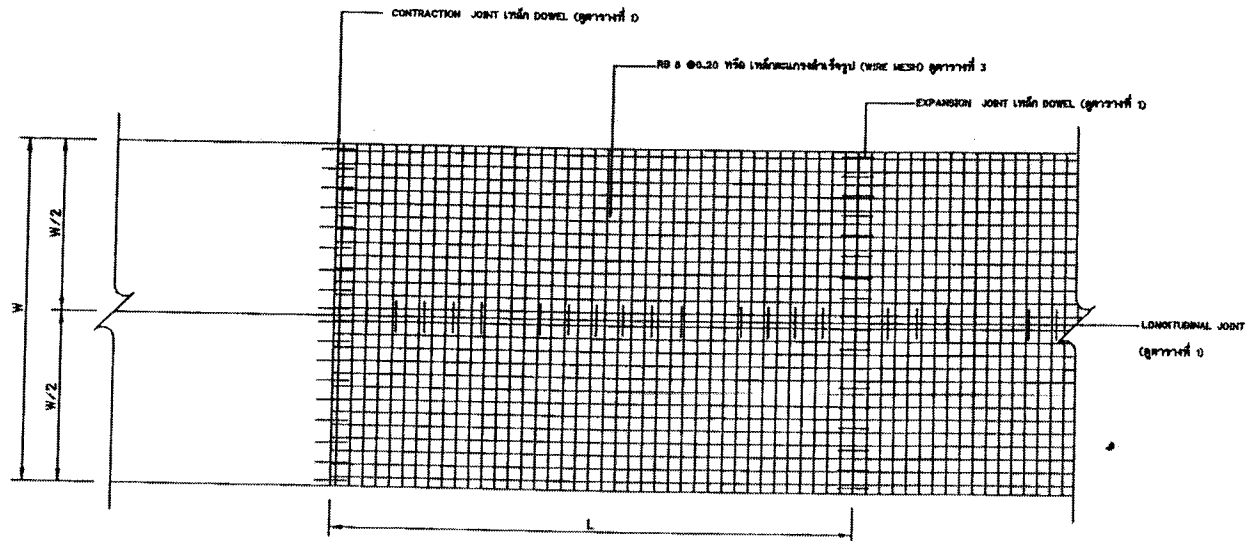
แบบแปลนแสดงการเสริมเหล็กถนน ค.ค.ค.
