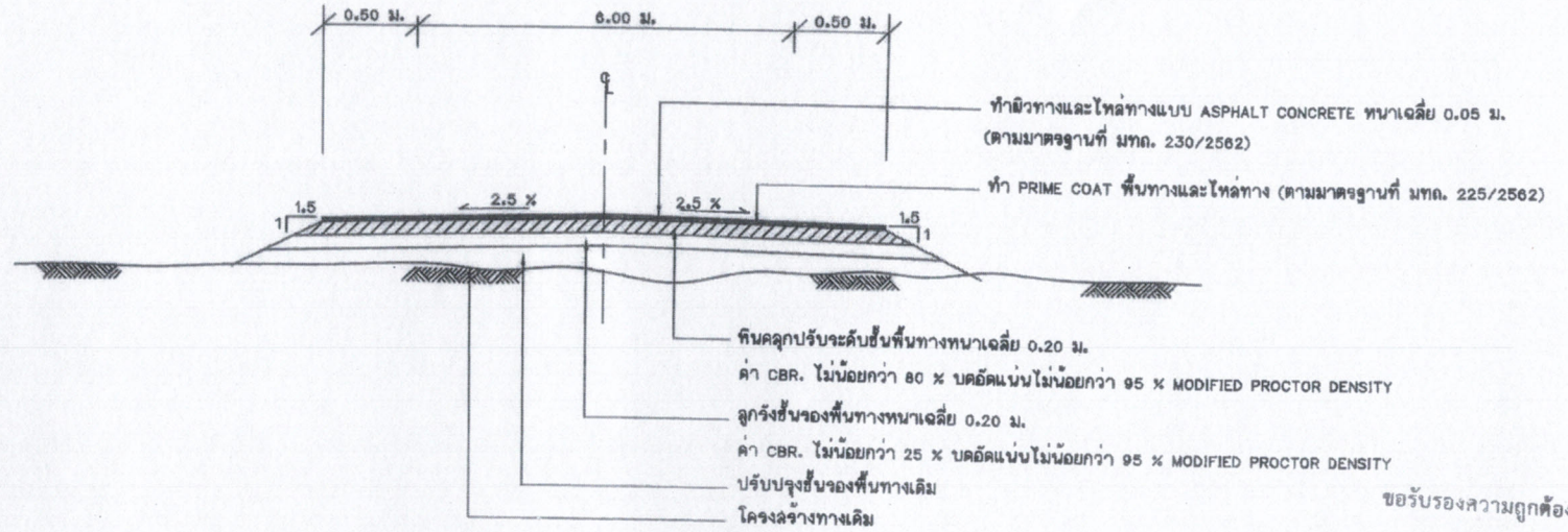
รูปตัดโครงสร้างทางผิวจราจรแบบ ASPHALT CONCRETE กม. 0+000 - กม. 1+000
