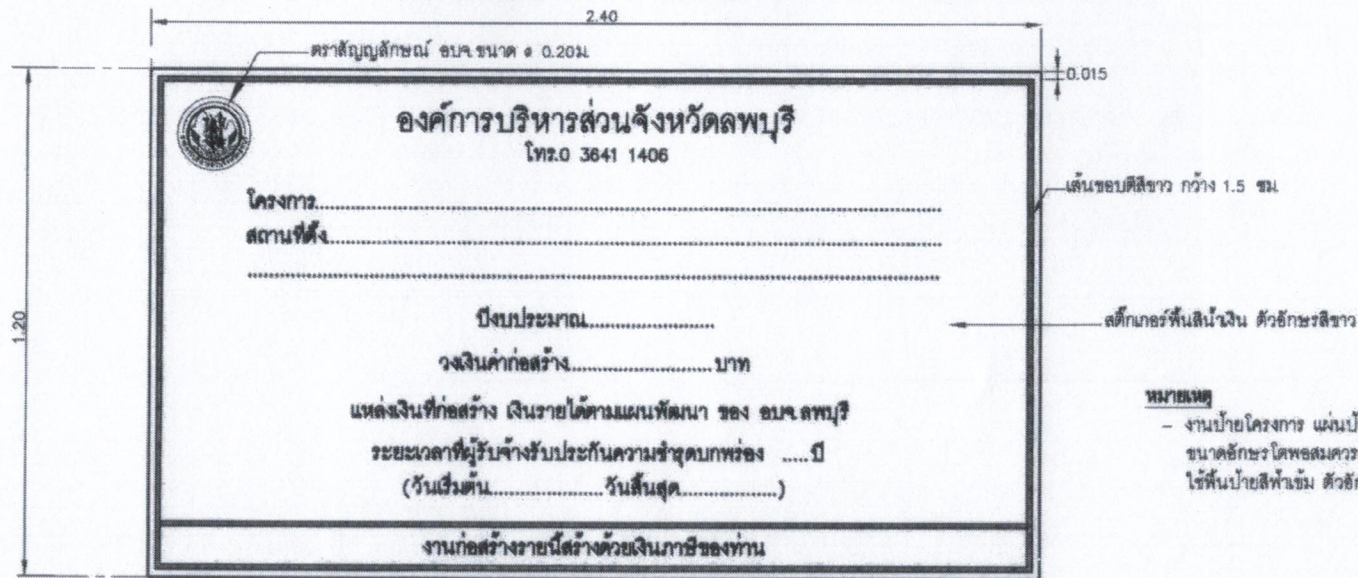
แบบขยายด้านหน้าแผ่นป้ายโครงการ
