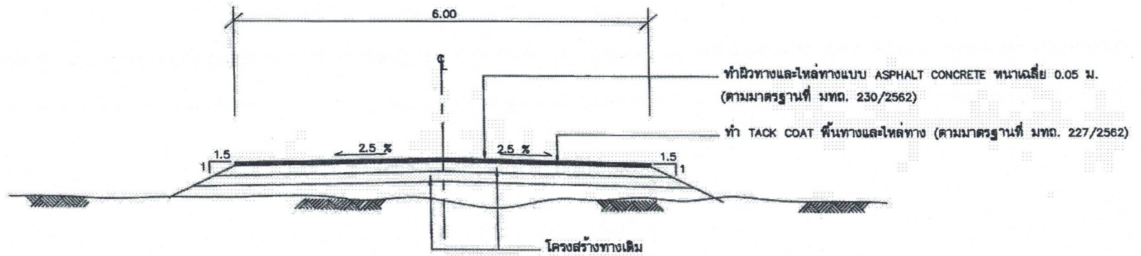
รูปตัดโครงสร้างทางผิวจราจรแบบ ASPHALT CONCRETE กม.ที่ 0+000 ถึง กม.ที่ 1+300
