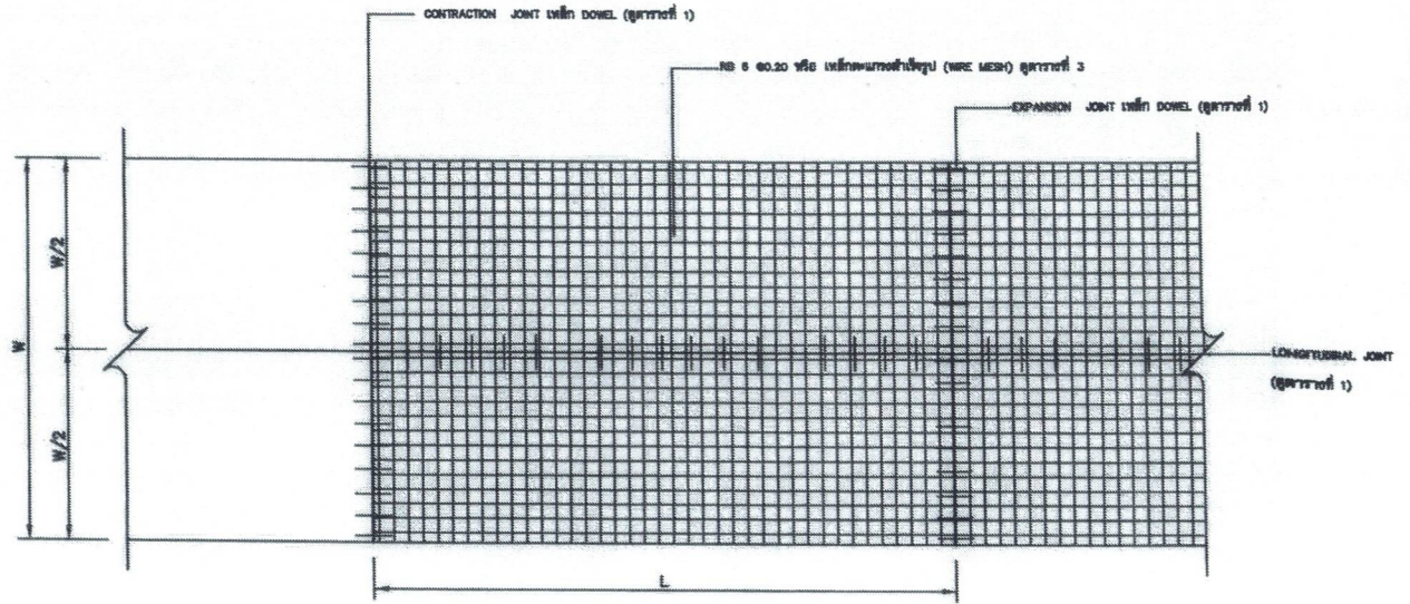
แบบแสดงการเสริมเหล็กถนน ค.ศ.ล.
