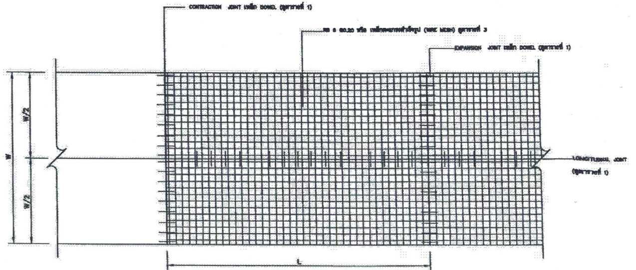
แบบแผนแสดงการเสริมเหล็กถนน ค.ศ.ศ.
