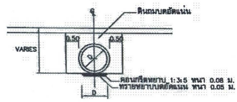
รูปตัดตามขวาง มาตรฐาน 1 : 100
