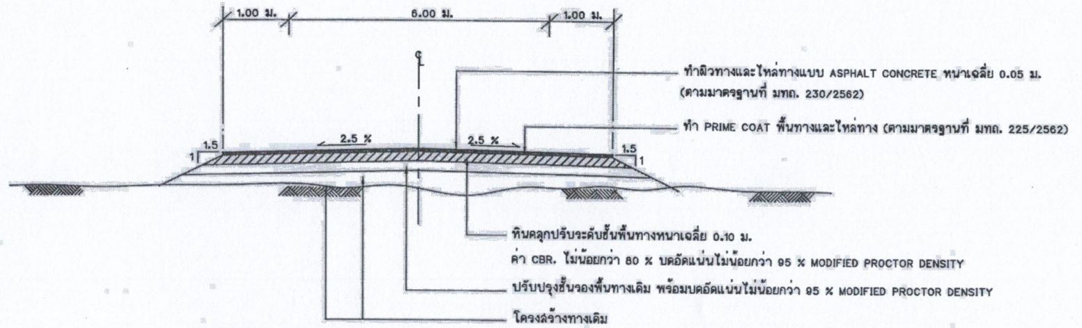
รูปตัดโครงสร้างทางผิวจราจรแบบ ASPHALT CONCRETE ช่วงที่ 1 กม.0+000 ถึง กม. 0+550
