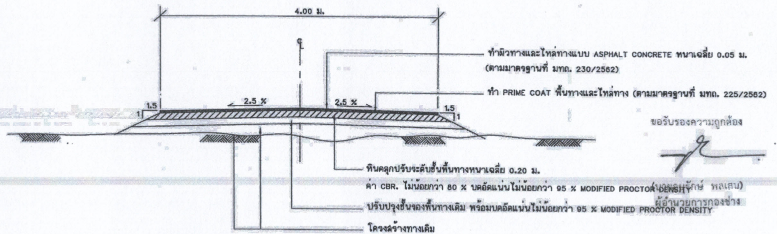
รูปตัดโครงสร้างทางผิวจราจรแบบ ASPHALT CONCRETE ช่วงที่ 2 กม.0+550 ถึง กม. 1+655
