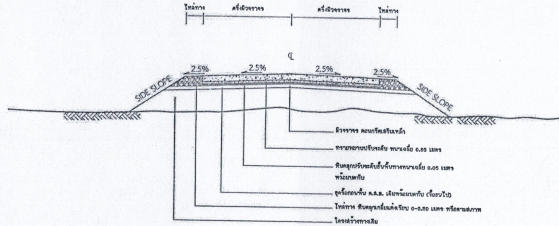
รูปตัดแฉ่งโครงการงานถนนคอนกรีตเสริมเหล็กและคูน้ำบ่อดีวีดี
