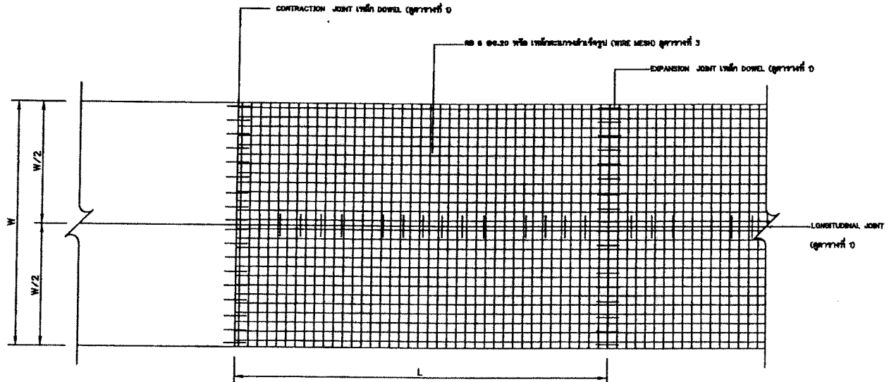
แบบแสดงการเสริมเหล็กถนน ค.ฉ.ล.
