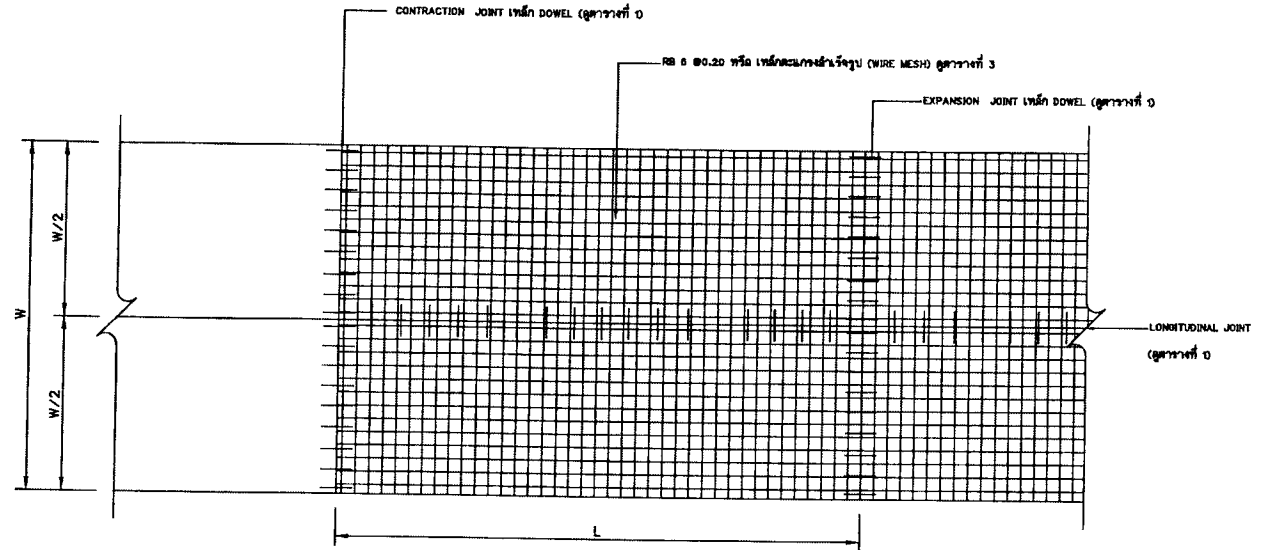
แปลนแสดงการเสริมเหล็กถนน ค.ฉ.ล.
