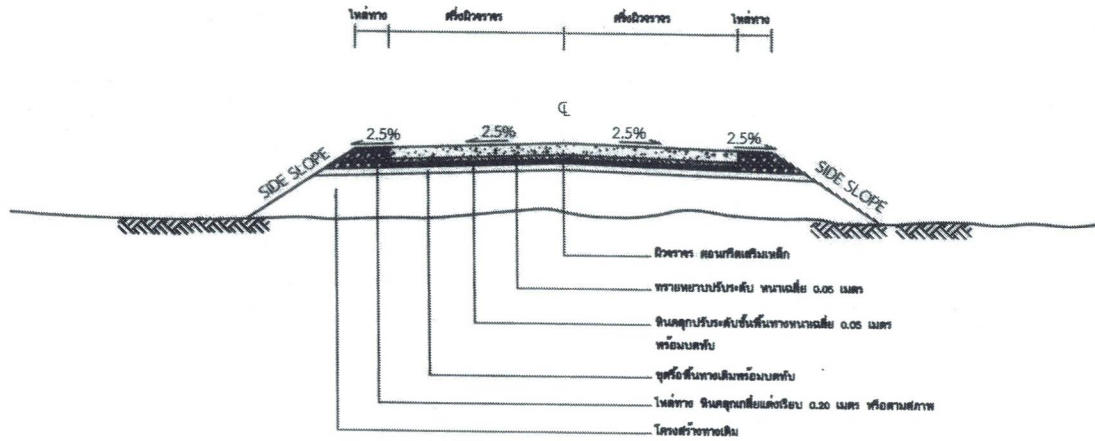
รูปตัดแสดงโครงสร้างถนนคอนกรีตเสริมเหล็กและคูผสมปิวี่สด
