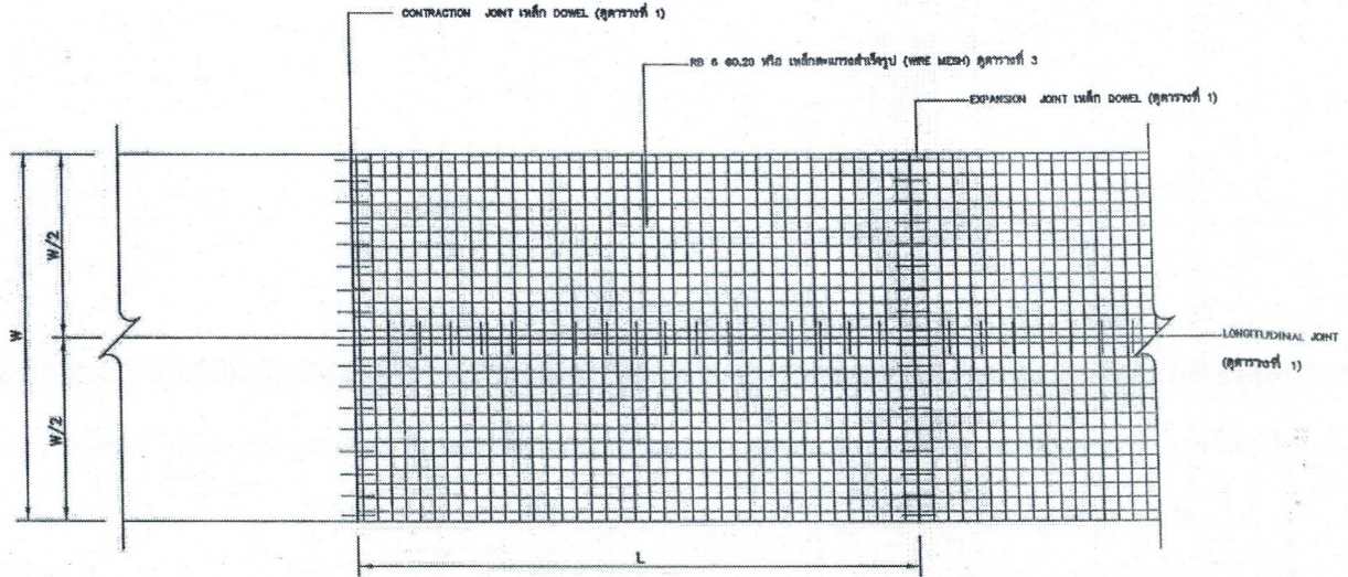
แปลนแสดงการเสริมเหล็กถนน ค.ศ.ล.
