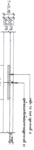
LONGITUDINAL JOINT
