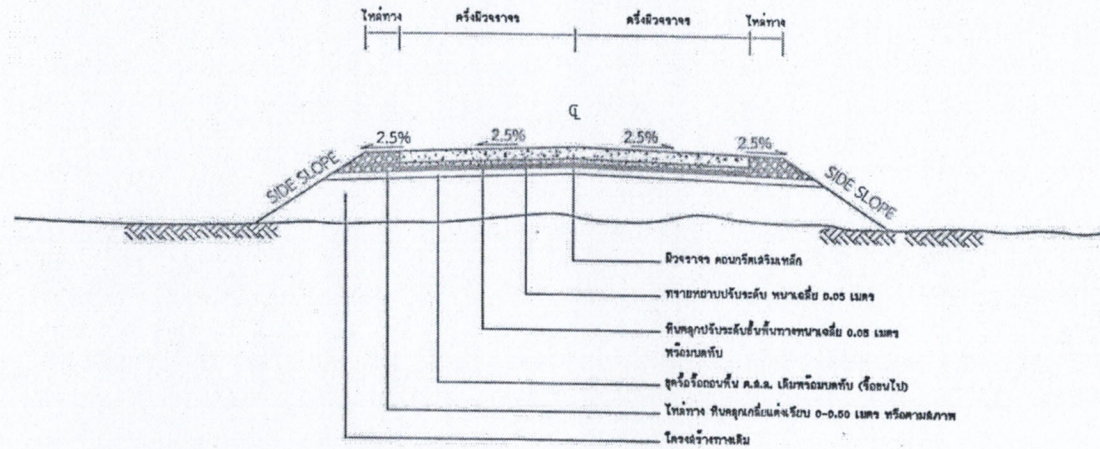
รูปตัดแฉะคงโครงค้ำฝังถนนคอนกรีตเสริมเหล็กและคูน้ำระบาย
