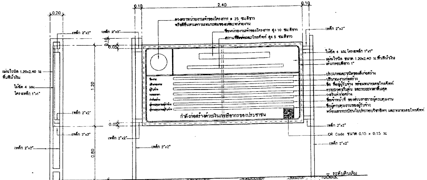
รูปด้านข้าง 1:20
