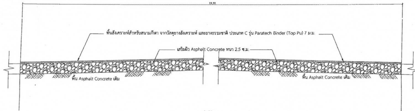
รูปตัด A-A มาตรฐาน 1:10
